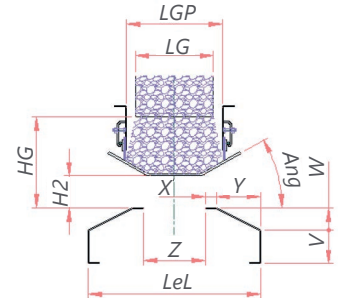
- Chasis C -
