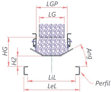
- Chasis A -
