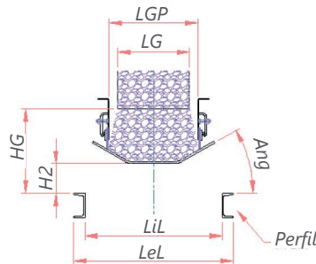
- Chasis B -
